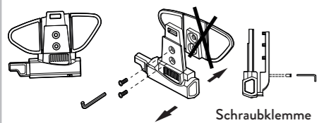
Schraubklemme
