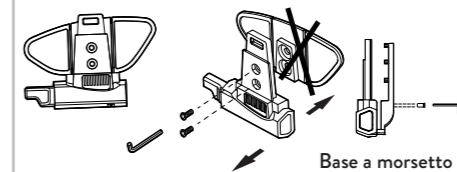
Base a morsetto
